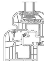
IDEAL 6000® (presek)
